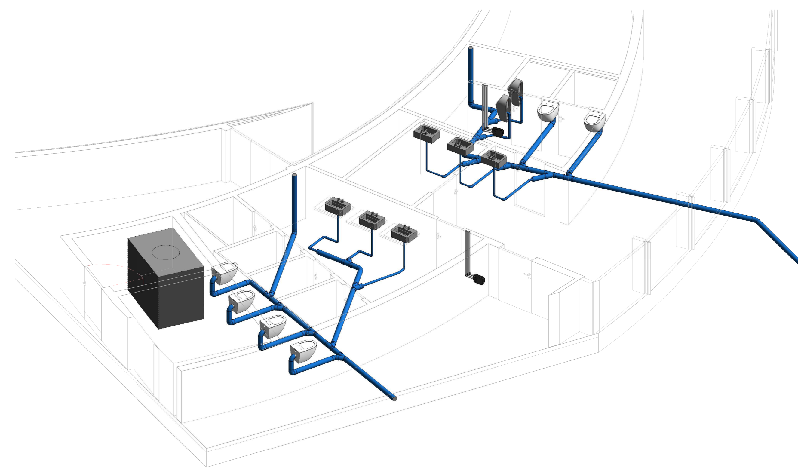
3 3D RETI DI SCARICO
