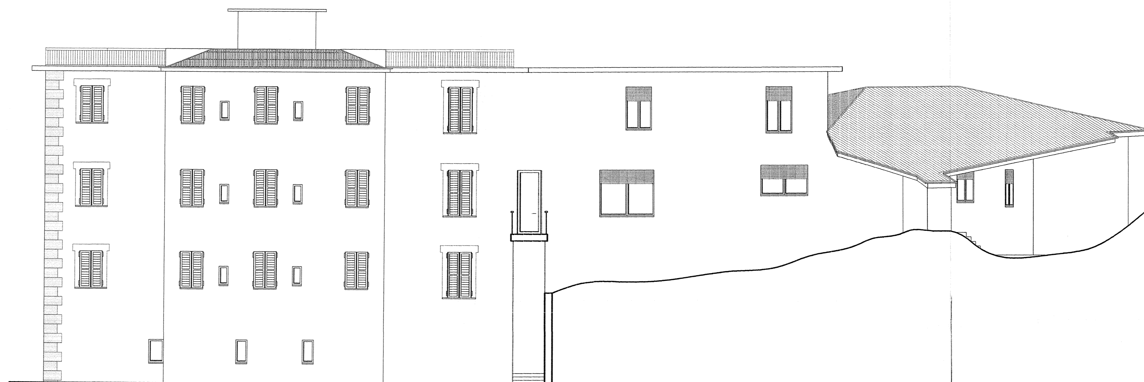
PROSPETTO OVEST - INTERNO
