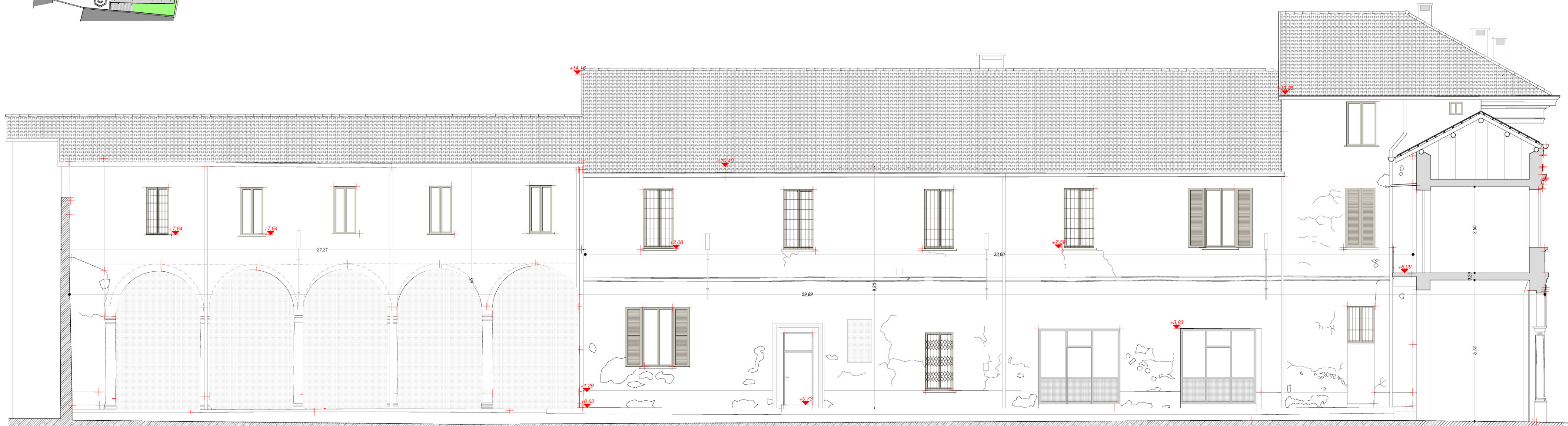
PROSPETTO CORTILE INTERNO LATO SUD - SEZIONE D-D
