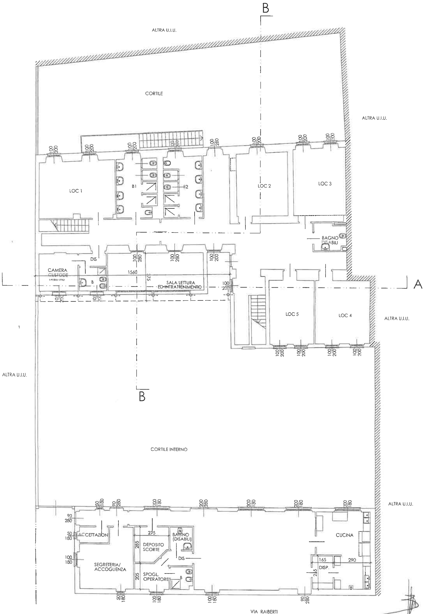
PIANTA PIANO TERRA - PROGETTO
